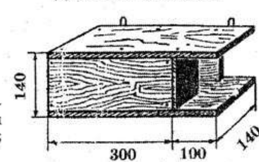
Домик для трясогузок
