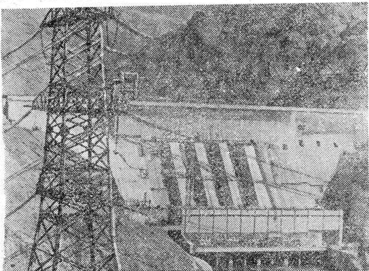
Курсайская ГЭС — четвертая на Нарынском каскаде. Она возведена в рекордно короткие сроки и полностью сдана в эксплуатацию в одиннадцатой пятилетке. Мощность станции — 800 тысяч киловатт.
