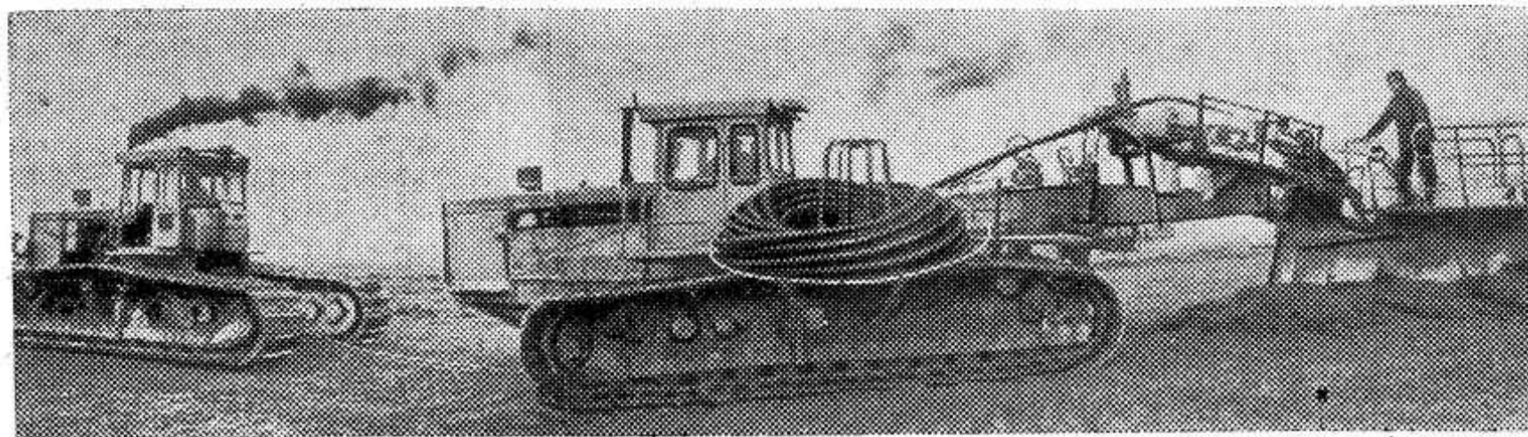
Смоленская область. Впервые на Смоленщине на землях совхоза имени Героя Советского Союза М. Егорова внедряется прогрессивный метод бестраншейной укладки дренажных полиэтиленовых труб (на снимке). Этот эффективный способ мелиоративного обустройства полей позволил значительно повысить производительность труда, высвободить часть техники, сэкономить десятки тонн горюче-смазочных материалов. (Фотохроника ТАСС).
