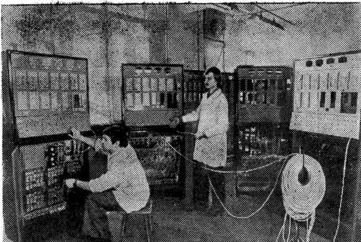
КАЗАХСКАЯ ССР. С конвейера Усть-Каменогорского завода приборы сошли первые пневматические управляющие машины — «ПУМ-1А», предназначенные для автоматизации процесса гранулирования кормов в животноводстве.
