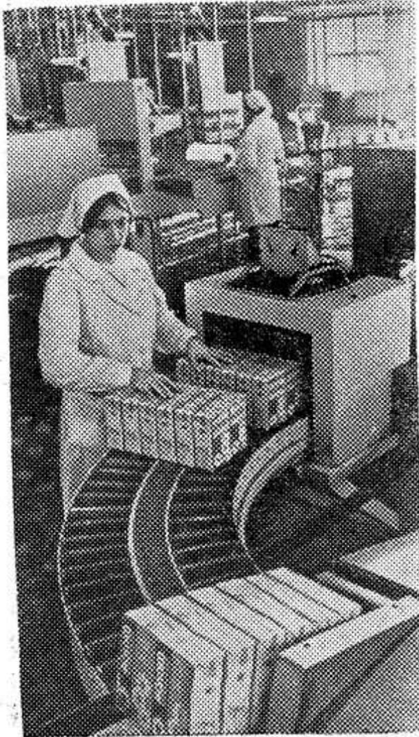
Московский молочный комбинат — крупнейшее в Европе автоматизированное предприятие. На нем люди только следят за работой сложных машин и агрега-
