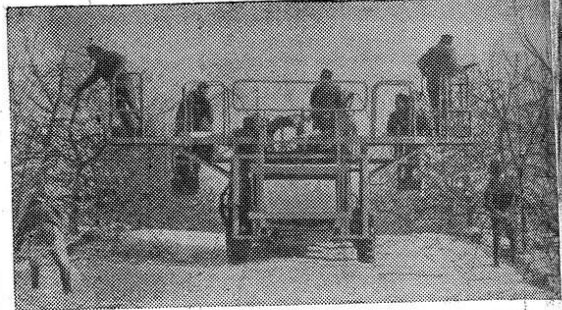
Венгрия. Этой весной на плантациях госхоза «Самошменти» подрезка более 200 тысяч яблоневых деревьев была проведена с помощью специальной техники. Самоходная пневматическая установка значительно облегчила трудоемкую операцию, выполнявшуюся раньше вручную. Фото МТИ — ТАСС.
