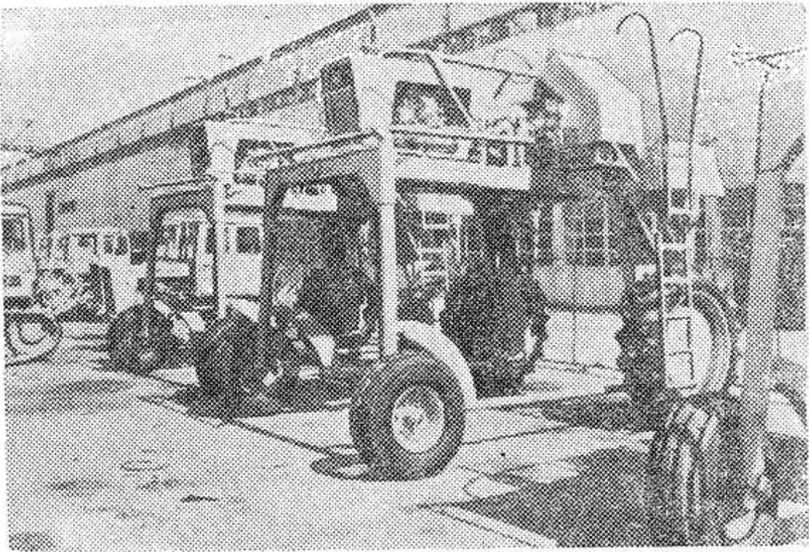
Болгария. Коллектив тракторного завода в городе Карлово приступил к выпуску новых виноградоуборочных комбайнов (на снимке), получивших во время испытания
