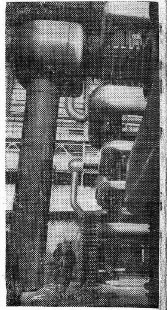
Запорожье. Во Всесоюзном научно-исследовательском институте трансформостроения построен самый крупный в стране зал для испытания трансформаторов. Сейчас идет монтаж технологического оборудования.
