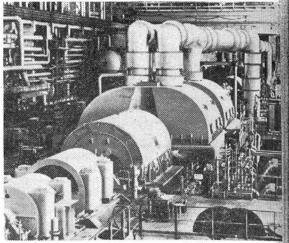
Турбинный зал атомной электростанции, сооружаемой близ Грейфсвальда на севере Германской Демократической Республики. Недавно здесь дат ток первый энергоблок мощностью 440 тысяч киловатт. Создание современной
