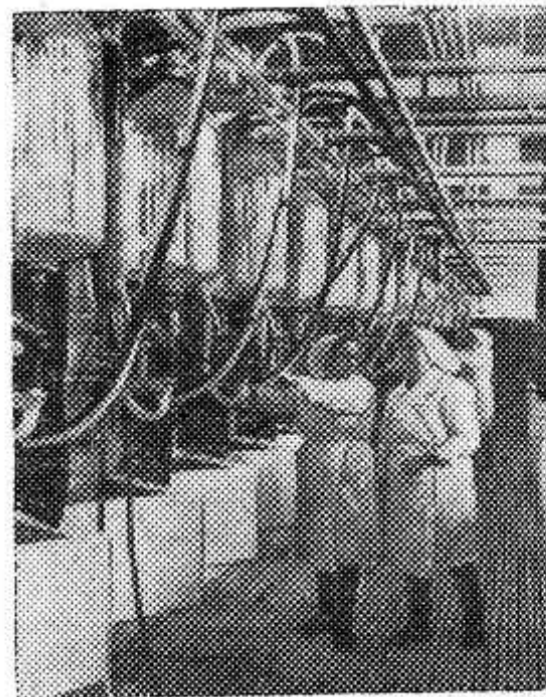
Ивано-Франковская область. В колхозе имени Ярослава Галана Косовского района сооружен молочный комплекс. Он состоит из механизированной фермы на 600 коров, доильного зала с установками типа «елочка», холодильных камер и кормоцеха.
