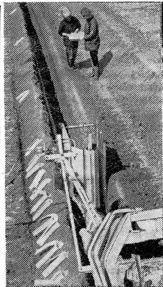
Ленинградская область. Лужская передвижная механизированная колонна управления «Ленмелиоводстрой» применяет поточно-комплексный метод мелиоративно-строительных работ, при котором все операции выполняются в строгой последовательности до полного завершения. Это позволило значительно повысить производительность труда механизаторов.
