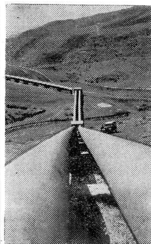
Армянская ССР. Для ороше... ния восьми тысяч гектаров зем... ли Ноемберянского района... сооружена многоступенчатая... насосная станция, которая... перекачивает воды реки Дебед... и дает живительную влагу садам... совхозов. Пять ступеней станции уже... действуют, строится шестая, по... следняя ступень, с помощью... которой вода будет поднята... на высоту 650 метров. Тогда... земельные угодья района будут... полностью обводнены. НА СНИМКЕ: по этому тру... бопроводу перекачиваются во... ды реки. Фото А. Агаджаняна.
