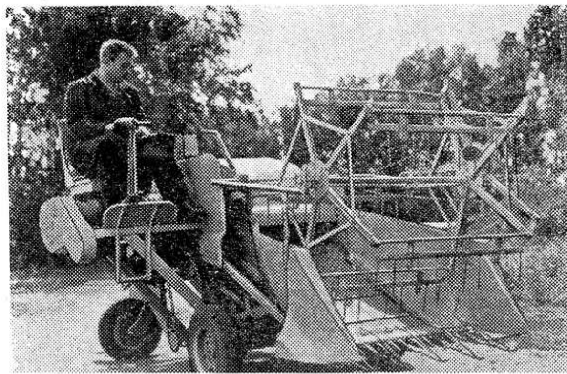
ОМСК. Коллектив опытного конструкторского бюро Сибирского научно-исследовательского института сельского хозяйства совместно с сотрудниками лаборатории механизации работ в селекции создали комплекс се-
