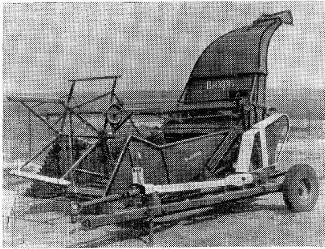
НА СНИМКЕ: прицепной силосоуборочный комбайн «Вихрь» (СК-18). Он имеет сменные рабочие органы — косилочные аппараты для нормального резания и для кукурузы, а также подборщик. Комбайн может работать с тракторами МТЗ-50, МТЗ-80, ДТ-50. Обслуживает его один тракторист. Производительность «Вихря» при ширине захвата 1,8 метра до 6,5 гектара в час.
