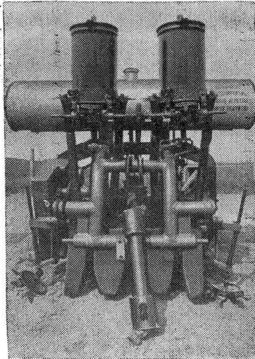
НА СНИМКЕ: агрегат по уходу за овощами АУО-1,4. Он выполняет одновременно операции по уничтожению сорняков, рыхлению почвы, внесению минеральных удобрений и обработке почвы гербицидами. Рабочая скорость агрегата на буксире трактора «Беларусь» — 7 километров в час. Обслуживается он трактористом.
