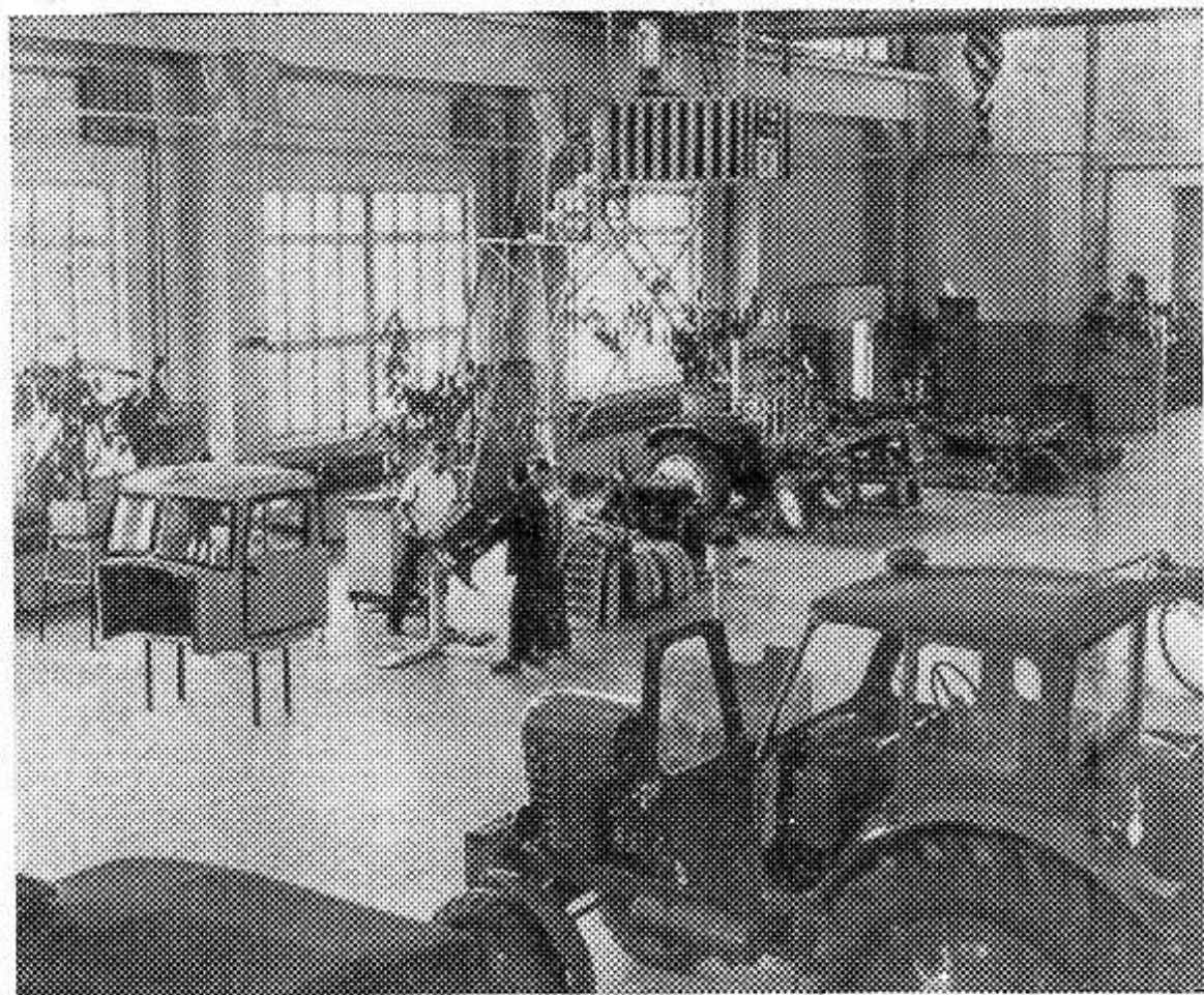
В лабораториях, на испытательных треках и полигонах Кубанского научно-исследовательского института испытаний тракторов и сельскохозяйственных машин проходят проверку, держат экзамен новые тракторы, самоходные шасси, комбайны, почвообрабатывающие навесные механизмы. Институт осуществляет научное руководство всеми машиноиспытательными станциями страны, разрабатывает методы и нормативы испытаний. Инженеры создали и усовершенствовали 345 стандов, различных приборов, испытательных установок. НА СНИМКЕ: в зале технической экспертизы тракторов. Фотохроника ТАСС.
