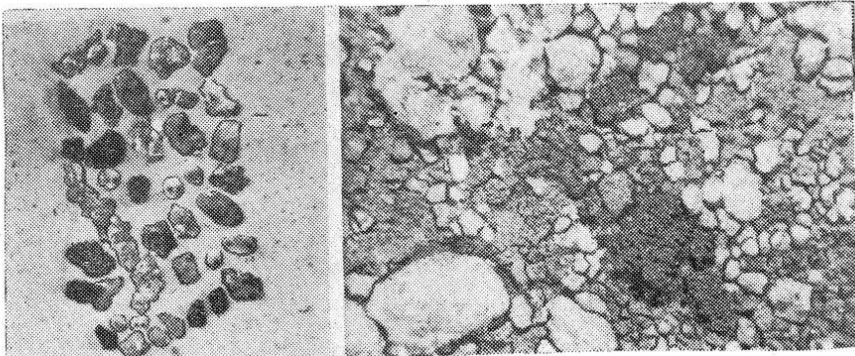
лунного грунта, доставленного автоматической станцией «Луна-16».
