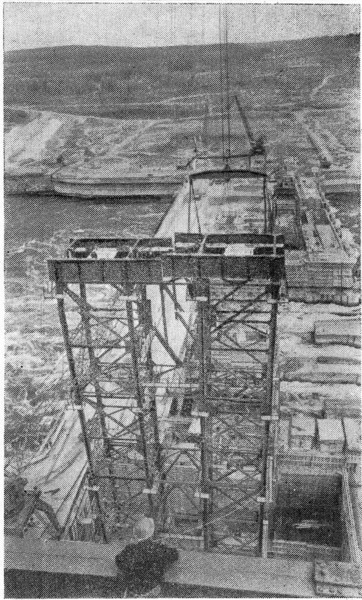
ИРКУТСКАЯ ОБЛАСТЬ. Полным ходом идет строительство Усть-Илимской ГЭС. Ведется подготовка к бетонированию плотины и фундамента под здание станции, монтируется большая бетоновозная эстакада, готовится к пуску второй, более мощный бетонный завод. С его пуском еще шире развернутся работы на сооружении энергетического гиганта. НА СНИМКЕ: монтаж большой бетоновозной эстакады. Фото М. Минеева. Фотохроника ТАСС.
