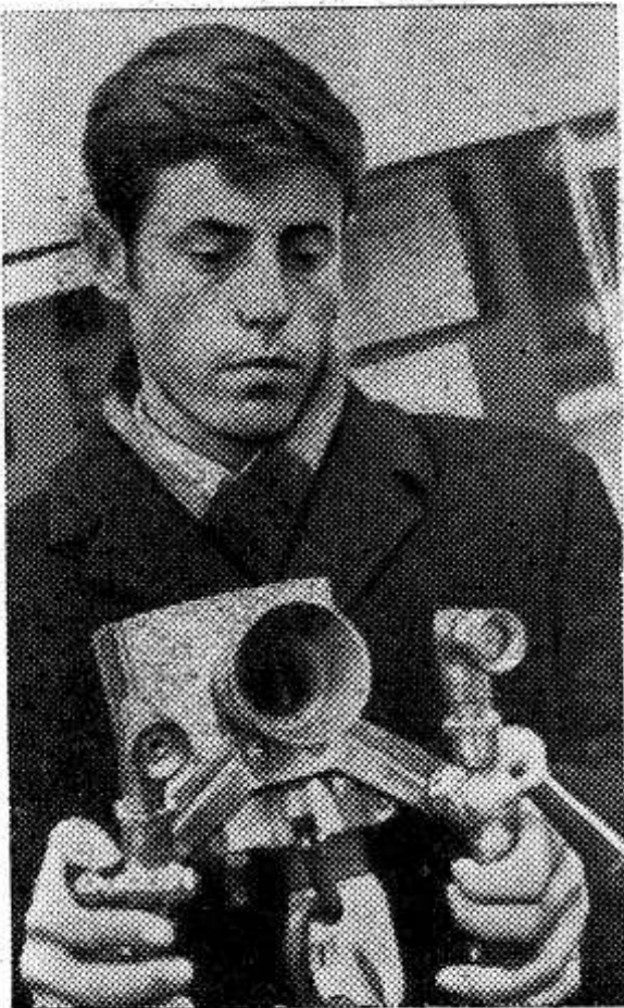
МОСКВА. Этот инструмент, позволяющий полностью механизировать процесс нанесения гидроизоляции при устройстве кровли, применяется строителями треста Калнинстрой № 1. Он закрепляется ремнями на груди рабочего и распыляет на обрабатываемую поверхность (любой формы) крошечный стекложгут, смоченный битумно-латексной эмульсией.
