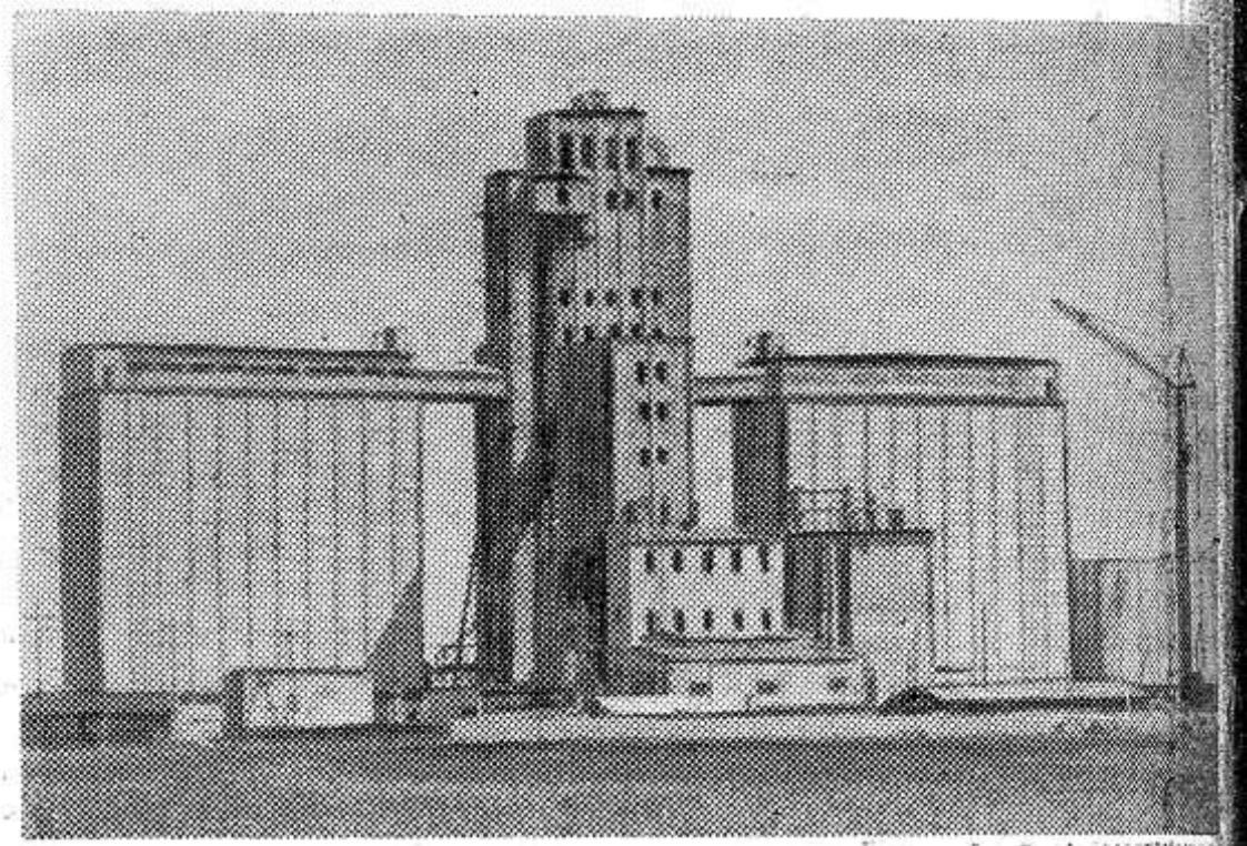
В селе Половинное Курганской области закончено строительство первой очереди крупнейшего в Зауралье элеватора (на снимке). Его силосные башни смонтированы из сборного железобетона. Весь процесс приемки, переработки и отгрузки зерна — автоматизирован. Фото С. Юдина. Фотохроника ТАСС.
