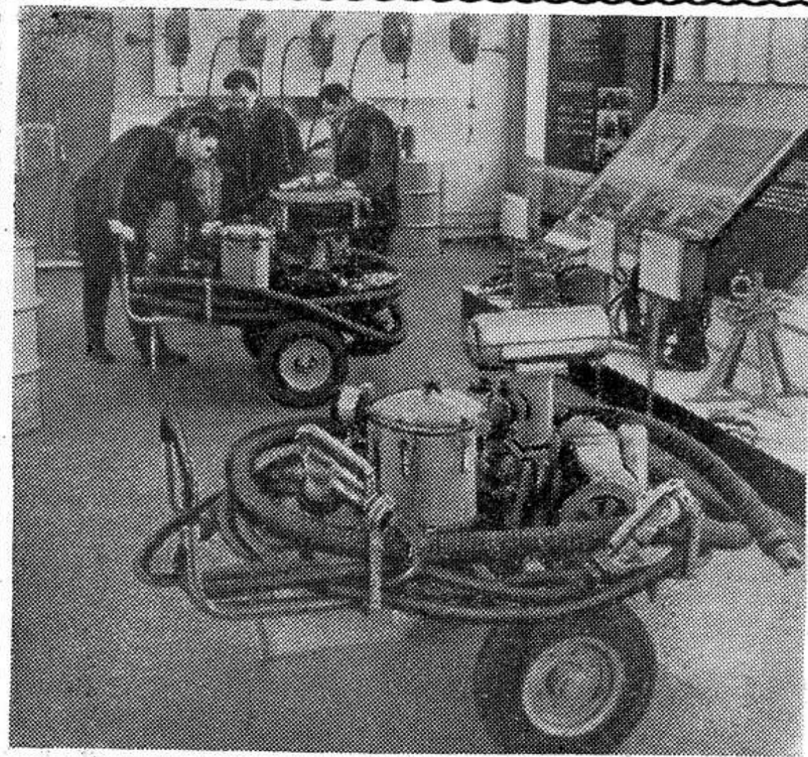
МОСКВА. В павильоне «Механизация и электрификация сельского хозяйства» ВДНХ СССР демонстрируются образцы современного оборудования, позволяющего свести до минимума потери горючих и смазочных материалов при заправке тракторов, комбайнов и автомобилей, в том числе — различные насосы для закрытой перекачки горючего из бочек в топливные баки машин в полевых условиях.
