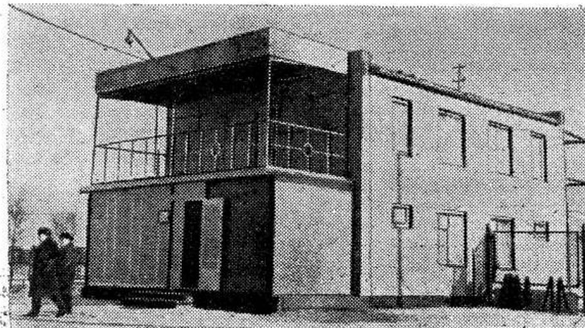
НА СНИМКЕ: образец жилого дома для сельской местности. Типовой двухэтажный дом на две семьи. Каждая квартира состоит из гостиной, детской, кухни, спальни, имеет балкон. Для строительства применяются блоки, облицовочные плиты, отделанные крошкой, и другие унифицированные детали. Фото В. Кунова. Фотохроника ТАСС.
