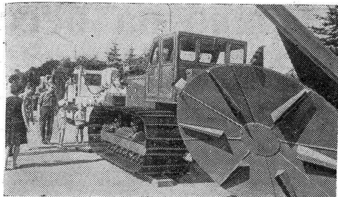
НА СНИМКЕ: фрезерный канавокопатель «КФП-1 200» Мозырского завода мелиоративных машин, предназначенный для прокладки осушительных каналов на торфяных грунтах глубиной от 0,65 до 1,2 метра и шириной по дну — 2,5 метра. Он навешивается на трактор «Т-100МБГС». Производительность — 260 кубометров в час. В этом году намечено выпустить 100 таких машин.
