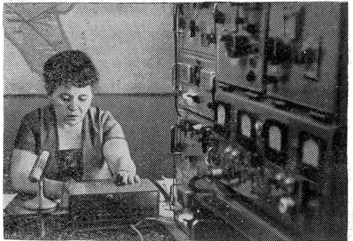
В Саратовской области организована диспетчерская служба сельского хозяйства. Непрерывная двухсторонняя радиосвязь со всеми районами области ликвидировала излишнюю переписку и разгрузила междугородную телефонную связь. Эта служба обеспечила оператив-
