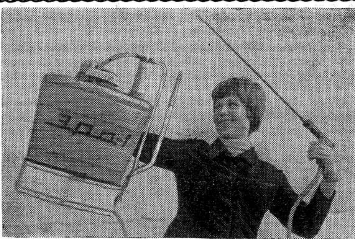
ХАРЬКОВ. «Эра-1» — переносной ручной опрыскиватель для химической борьбы с вредителями виноградников и садов, расположенных в труднодоступных местах, где нет возможности применить более производительные машины, — изготовлен Украинским научно-исследовательским институтом сельскохозяйственных машин совместно с Львовским ГСКБ по машинам для химической защиты растений.
