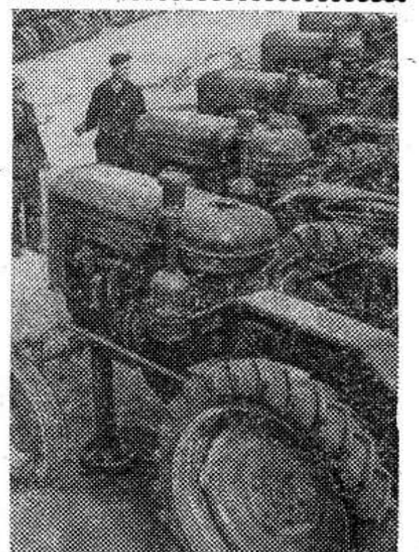
—КИРГИЗСКАЯ ССР. Круглогодичный ремонт машинно-тракторного парка организован в Московском районном объединении «Киргизсельхозтехника». Прогрессивный поточный метод ремонта и обменный фонд тракторов обеспечивают бесперебойную работу колхозных и совхозных парков Чуйской долины.
