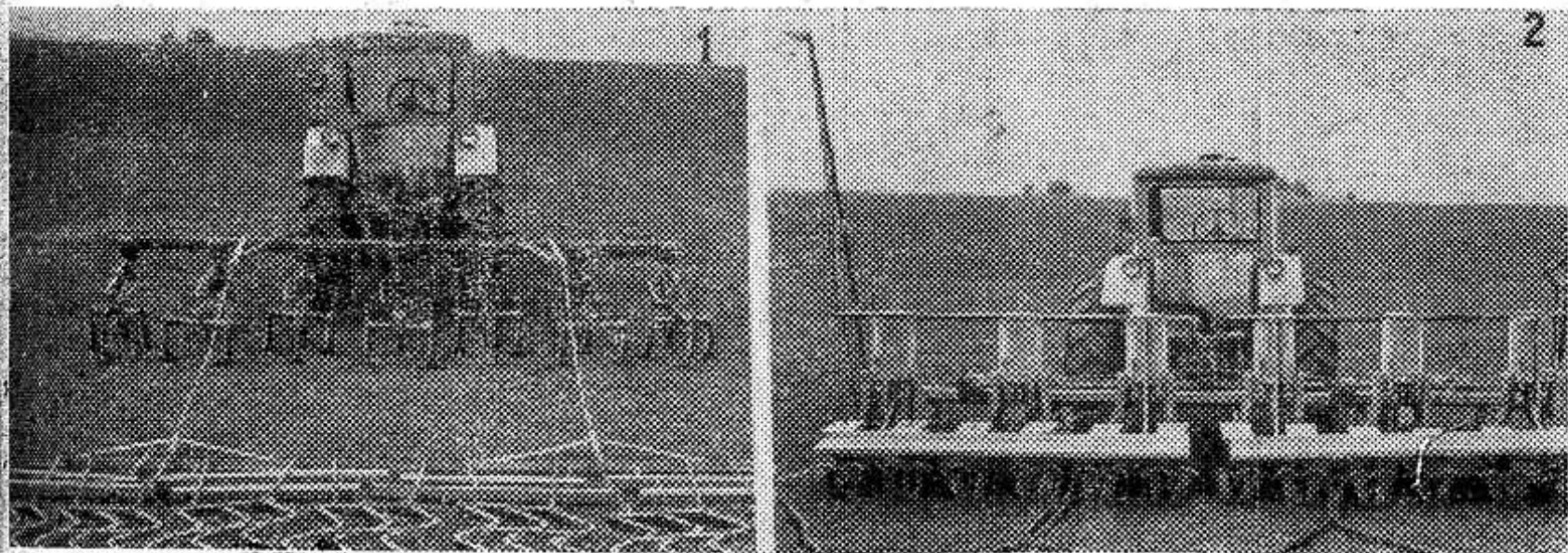
Курская область. На Центрально-черноземной машиноиспытательной станции проводятся испытания механизмов для обработки плантаций сахарной свеклы. На снимках: машины универсальной системы (УСМО-12): 1 — культиватор КРН-4,2 для предпосевной обработки почвы. 2 — двенадцатирядная сеялка. Фото О. Сизова. Фотохроника ТАСС.
