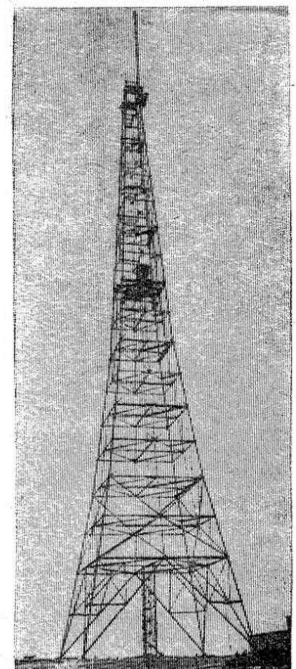
В селе Глубокое ведутся работы по установке радиорелейной вышки. Она уже поднялась на 155 метров. Сборка конструкций сейчас производится готовыми секциями, что намного ускоряет строительство. Одновременно монтажники устанавливают на вышке необходимое оборудование для приема и ретрансляции телевизионных передач. Июль — месяц основных работ по монтажу.
