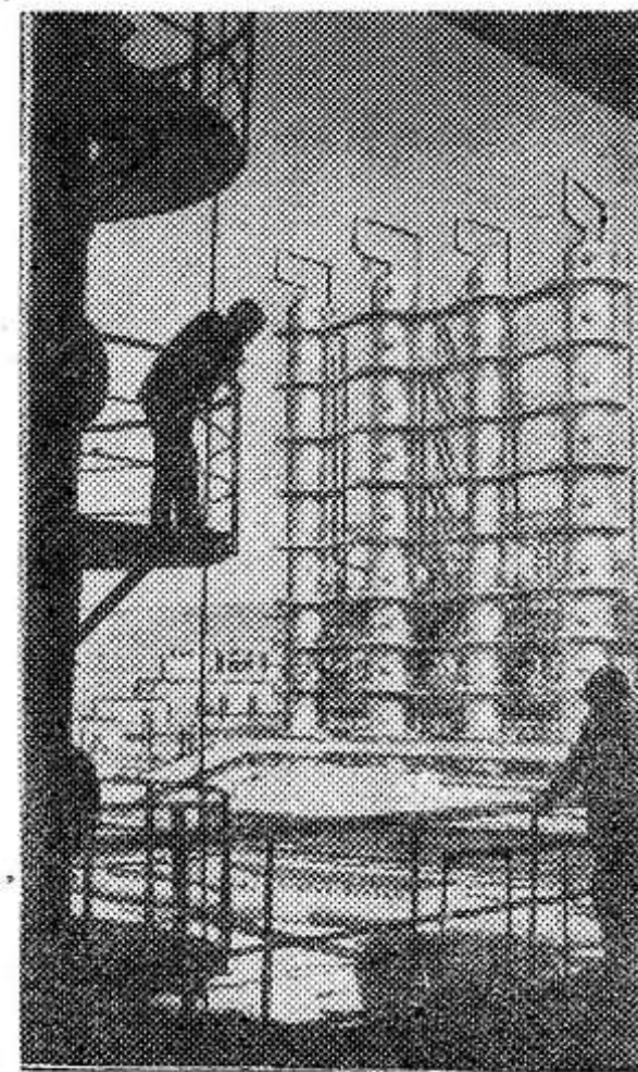
Ереван. Отделение ректификации завода «Поливинилцелат».
