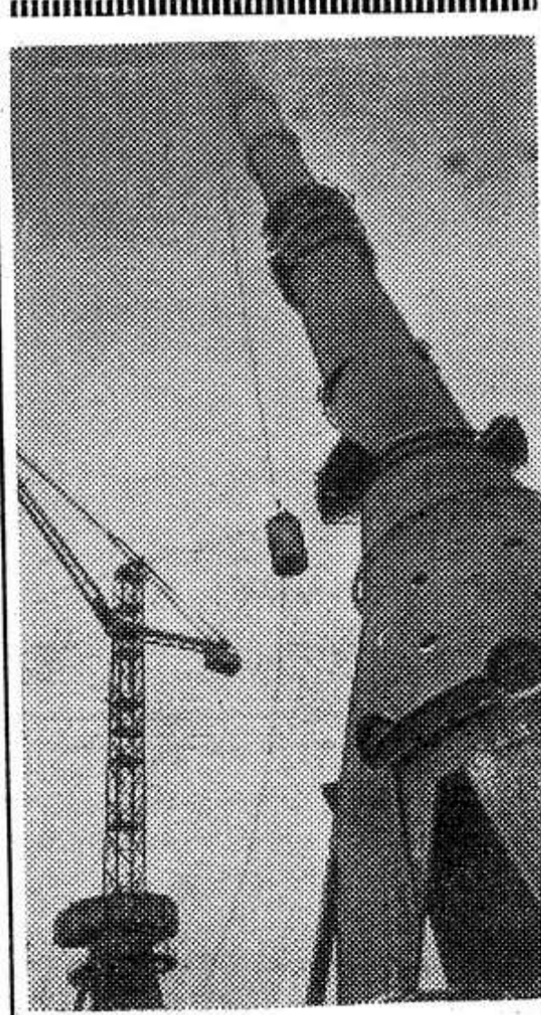
МОСКВА. Монтажники Опочечкинской телевизионной башни произвели подъем первой 23-тонной секции, являющейся основанием металлической антенны, которой увенчается высочайшая башня мира. Поднята также вторая секция. После подъема остальных частей антенны высота телебашни достигнет 533 метров. На снимке: подъем секции. Фото А. Стужина.
