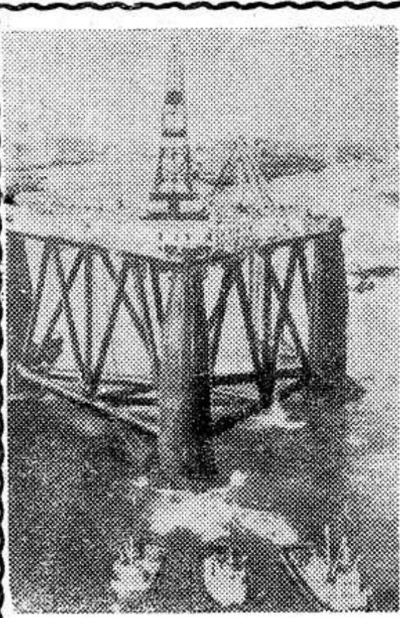
Искусственный английский остров «Си Квест» перемещается из лондонского порта к месту изыскательных работ в Северном море. С поверхности этого острова можно вести исследования глубин морей и океанов и использовать природные богатства, скрытые под водой на глубине 7.000 метров. Высота острова 115 метров, на нем может разместиться 60 человек. Фото ЧТК—ТАСС.
