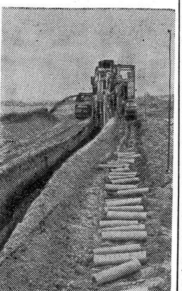
НОВГОРОДСКАЯ ОБЛАСТЬ. Более 250 гектаров земель будет осушено в нынешнем году в колхозе «Заря» Старорусского района. Осушение ведется методом закрытого дренажа при помощи высокопроизводительных механизмов.
