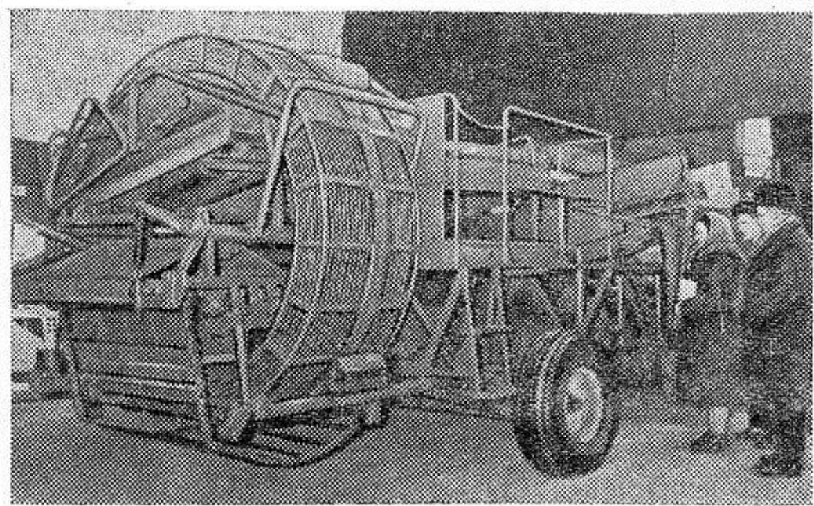
МОСКВА. На территории ВДНХ СССР открыта большая тематическая выставка, посвященная мероприятиям по подъему экономики сельского хозяйства нечерноземной зоны СССР. Одна из новинок, представленных здесь,—картофелеуборочный комбайн «ККУ-2», сконструированный сотрудниками ярославского Головного специализированного конструкторского бюро по машинам для возделыва-
