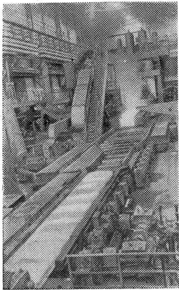
Один из крупнейших в мире автоматизированный блюминг «1300», вступивший в эксплуатацию на Челябинском металлургическом заводе, уже дал тысячи заготовок для электропрокатных станов. Оборудование технологической линии работает безупречно. Трудовую вахту у приборов управления несут лучшие прокатчики.
