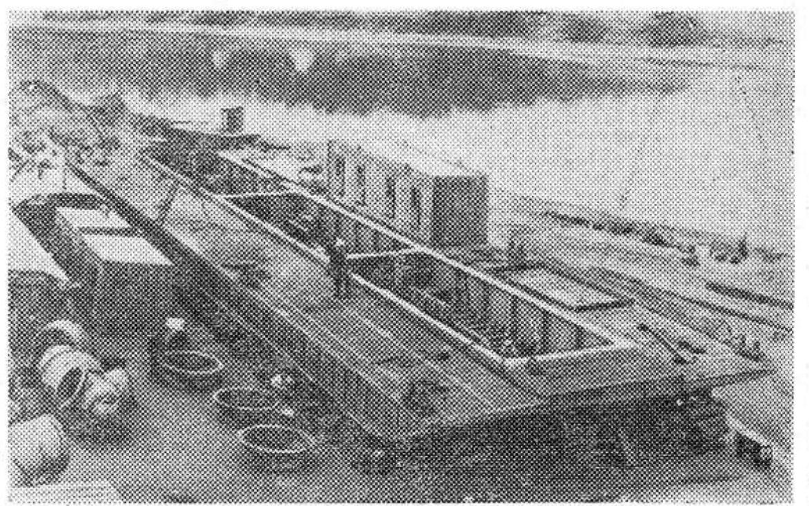
Коллектив Северочешского завода «Чешские судоверфи» изготавливает по заказу Советского Союза плавучие насосные станции, предназначенные для оро-
