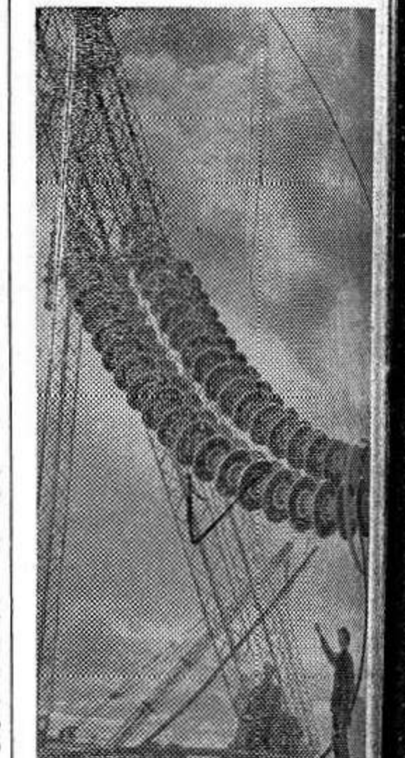
ПЕРМСКАЯ ОБЛАСТЬ. Строители Воткинской ГЭС ведут монтаж мощной открытой распределительной установки на 500 киловольт. Монтажники-высотники протягивают электротранзит от здания трансформаторной к береговому опору. Эту работу они стремятся завершить досрочно.
