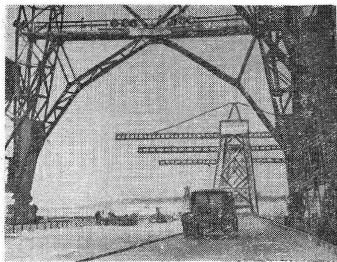
ИРКУТСКАЯ ОБЛАСТЬ. Ни днем, ни ночью не затихает гул гигантской стройки. Коллектив гидростроителей Братской ГЭС прилагает усилия к тому, чтобы сократить сроки монтажа оборудования. НА СНИМКЕ: на главной бетонной эстакаде. Фото Н. Перка.
