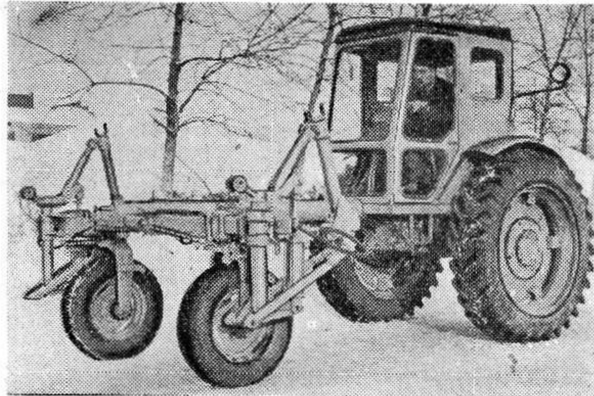
На Липецком тракторном заводе сконструировано самоходное шасси «СШ-40» для возделывания пропашных культур, главным образом сахарной свеклы (мощность двигателя 40 ло-
