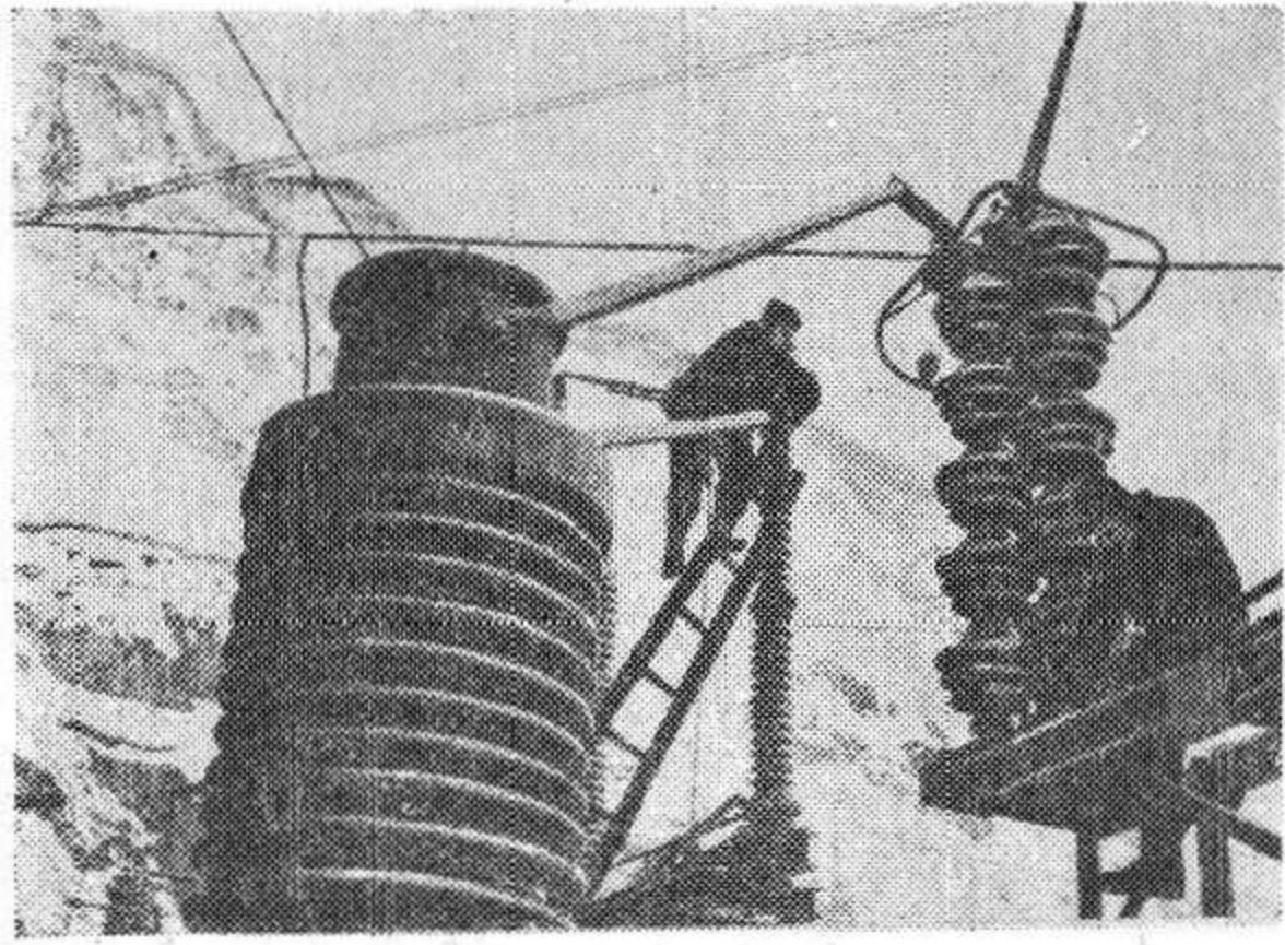
ВОСТОЧНО-КАЗАХСТАНСКАЯ ОБЛАСТЬ. Строители Бухтарминской ГЭС получили от уральцев уникальные автотрансформаторы. Их установка позволит давать дешевую энергию отдаленным потребителям Семипалатинской области и Алтайского края. НА СНИМКЕ: монтаж открытого распределительного устройства на 220 киловольт. Фото Ф. Сальникова. Фотохроника ТАСС.
